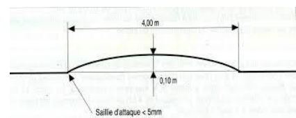
Profil en long ralentisseur dos d'âne
